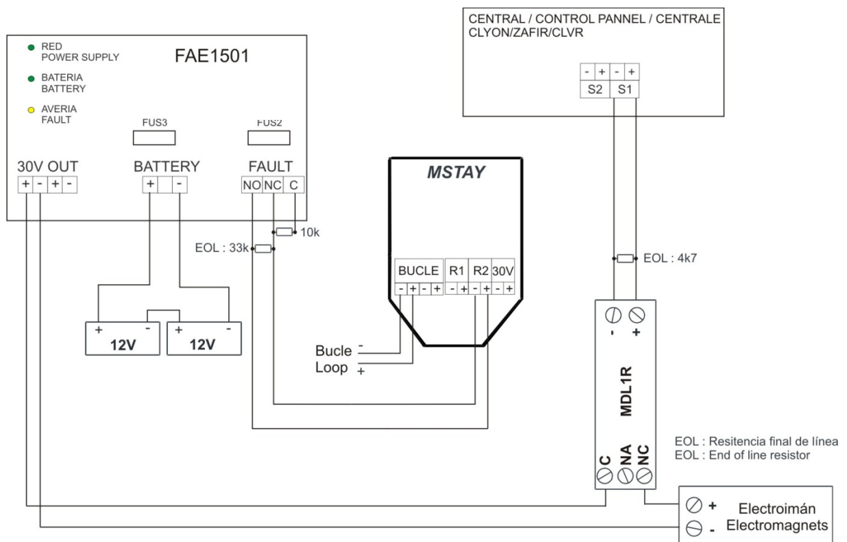
Figure 2: Schéma de câblage de sortie d'averie
