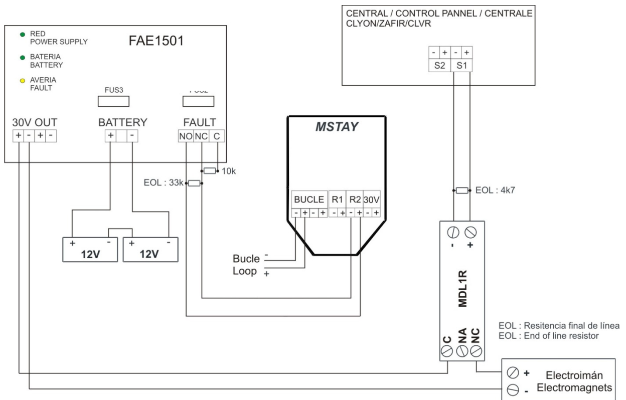
Figura 2: Esquema conxionado salida de avería
